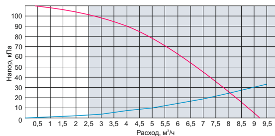
OD-40.0-50-120-P3-WL
