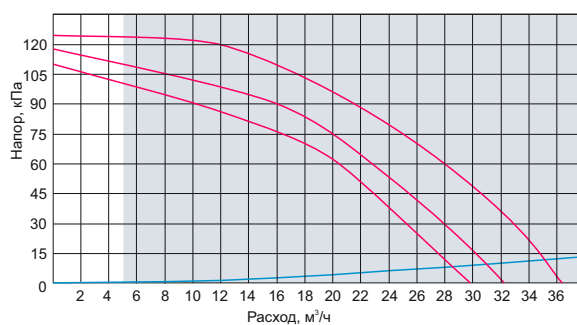
OD-90.0-80-120-P3-GL
