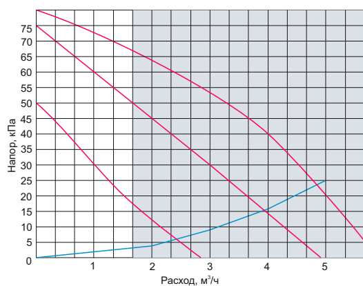
OD-10.0-32-80-P1-GL
