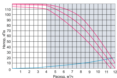
OD-25.0-40-120-P3-GL
