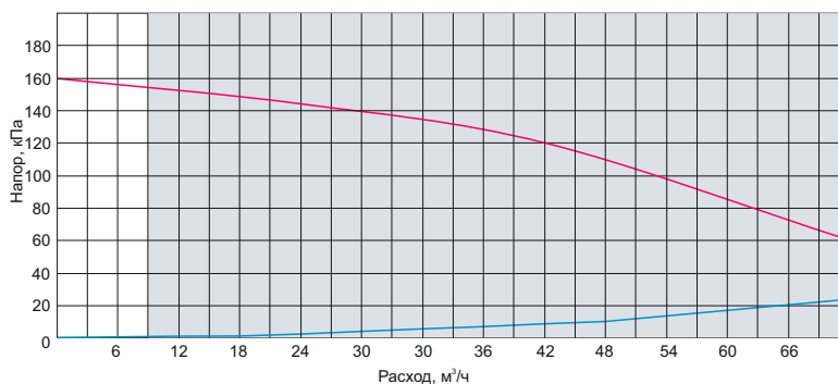
OD-150.0-100-160-P3-GL
